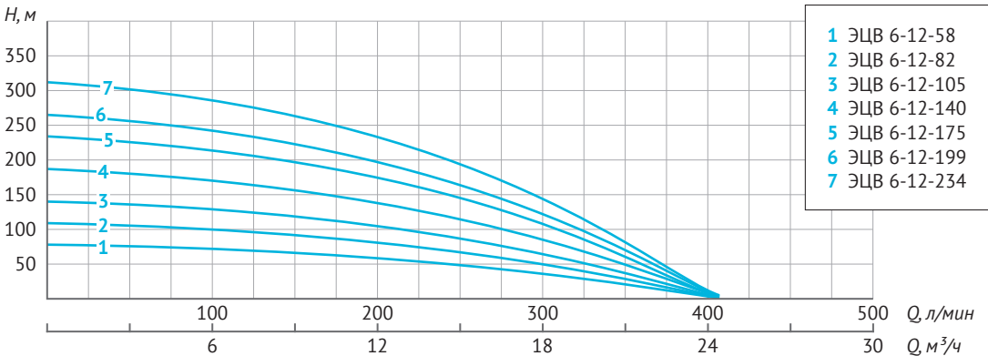
Напорно-расходные характеристики
